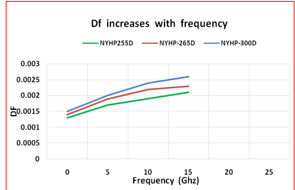
Df 与频率的关系 Df vs. Frequency
